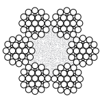
6 x 25 Filler Wire
