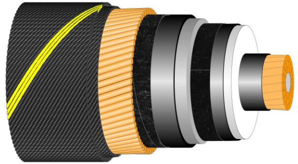
Resim 1: Asya-Avrupa bağlantısını sağlayan Türkiye'nin ilk 380 kV 1600 mm 2 kesitli Denizaltı Yüksek Gerilim Enerji Kablosu
